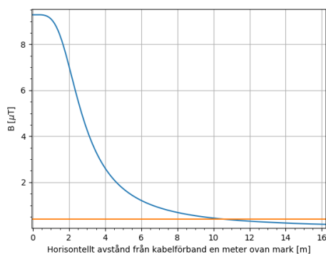
Figur 3. Magnetfältets utbredning för årsmedelvärde mellan område 4 och transformatorstationen vid anslutningspunkten. Magnetfältets storlek understiger 0,4 \mu\text{T} vid ca 11 m från kabelförbanden.
