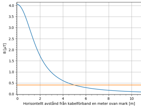
Figur 1. Magnetfältets utbredning för årsmedelvärde mellan område 1 och 2 i Bilaga 2. Magnetfältets storlek understiger 0,4 \mu\text{T} vid ca 5 m från kabelförbanden.
