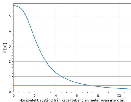
Figur 5. Magnetfältets utbredning för årsmedelvärde mellan område 7 - 6. Magnetfältets årsmedelvärde understiger 0,4 \mu\text{T} vid ca 8 m från kabelförbanden.
