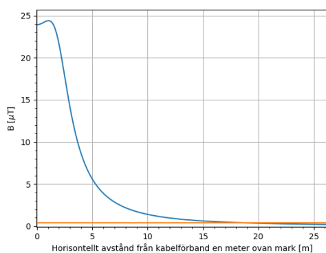
Figur 7 Magnetfältets utbredning från sex kabelförband som är anslutna till transformatorstationen vid anslutningspunkten beräknat för nominell ström 420 A. Magnetfältets storlek understiger 0,4 \mu\text{T} vid ca 20 m från kabelförbanden vid transformatorstationen.
