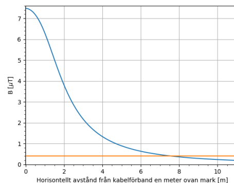
Figur 4. Magnetfältets utbredning för årsmedelvärde mellan område 6 och transformatorstationen vid anslutningspunkten. Magnetfältets storlek understiger 0,4 \mu\text{T} vid ca 8 m från kabelförbanden.
