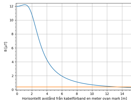
Figur 6. Magnetfältets utbredning från sex kabelförband som är anslutna till transformatorstationen vid anslutningspunkten beräknat för strömmens årsmedelvärde. Magnetfältets årsmedelvärde understiger 0,4 \mu\text{T} vid ca 14 m från kabelförbanden.
