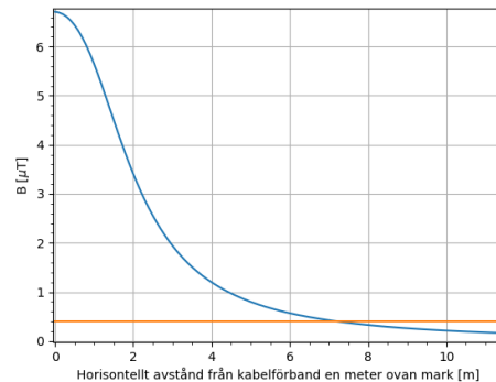
Figur 2. Magnetfältets utbredning för årsmedelvärde mellan område 2, 3 och 4. Magnetfältets storlek understiger 0,4 \mu\text{T} vid ca 7 m från kabelförbanden.
