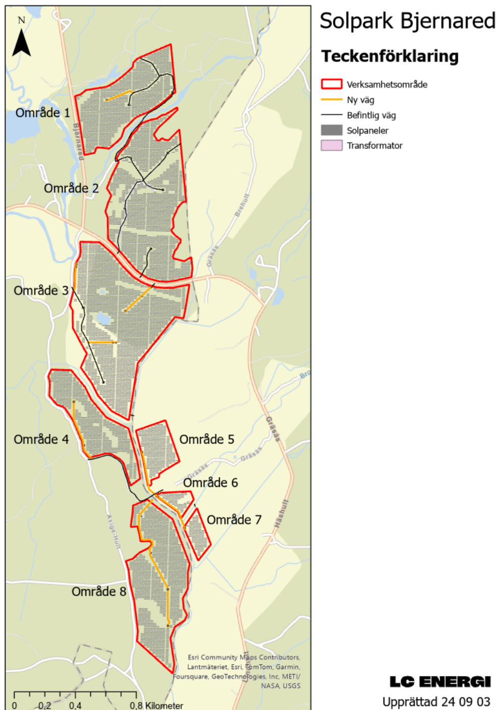
Figur 3. Exempellayout (källa: LC Energi)
