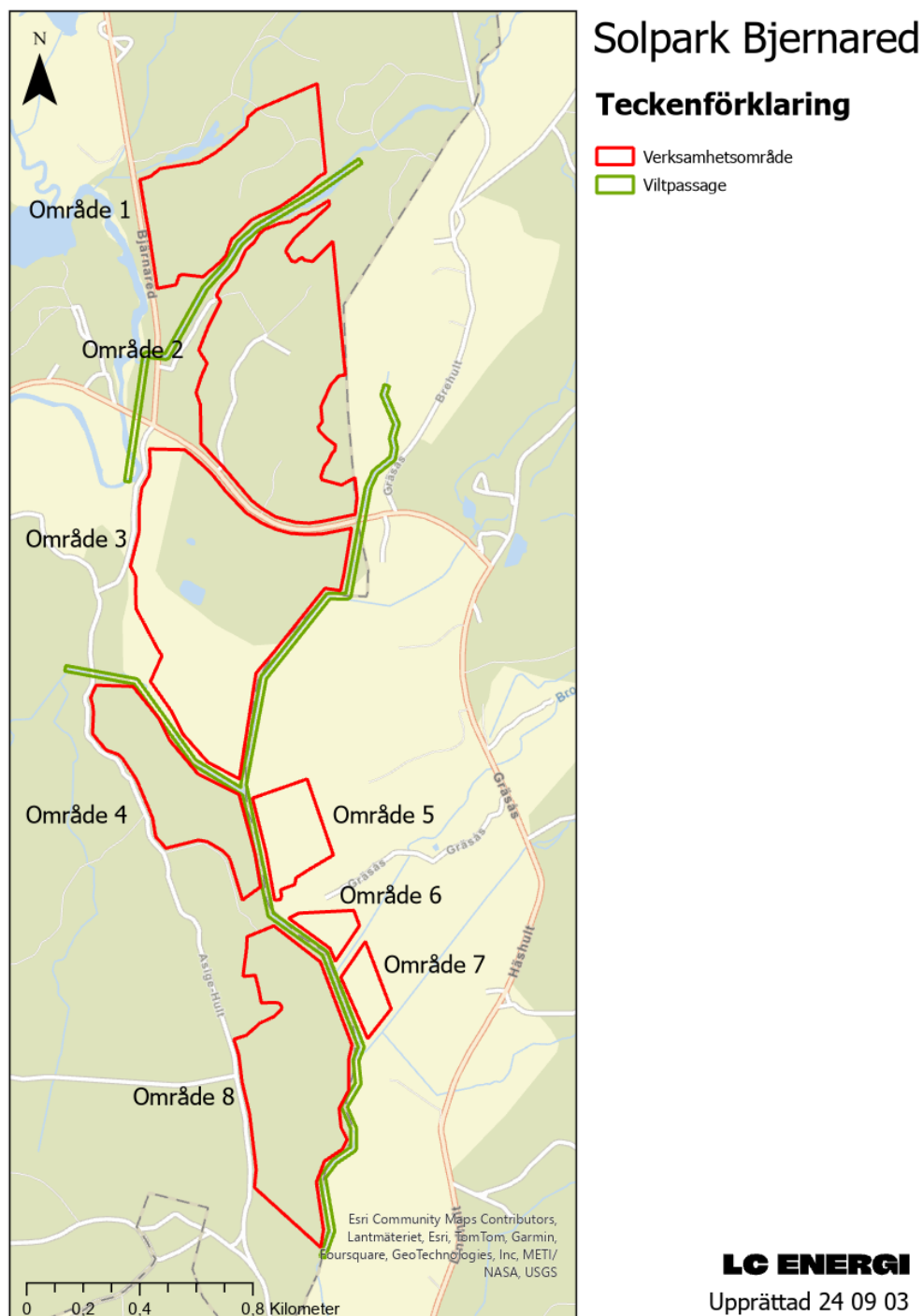
Figur 17. Viltpassager. (LC Energi)
