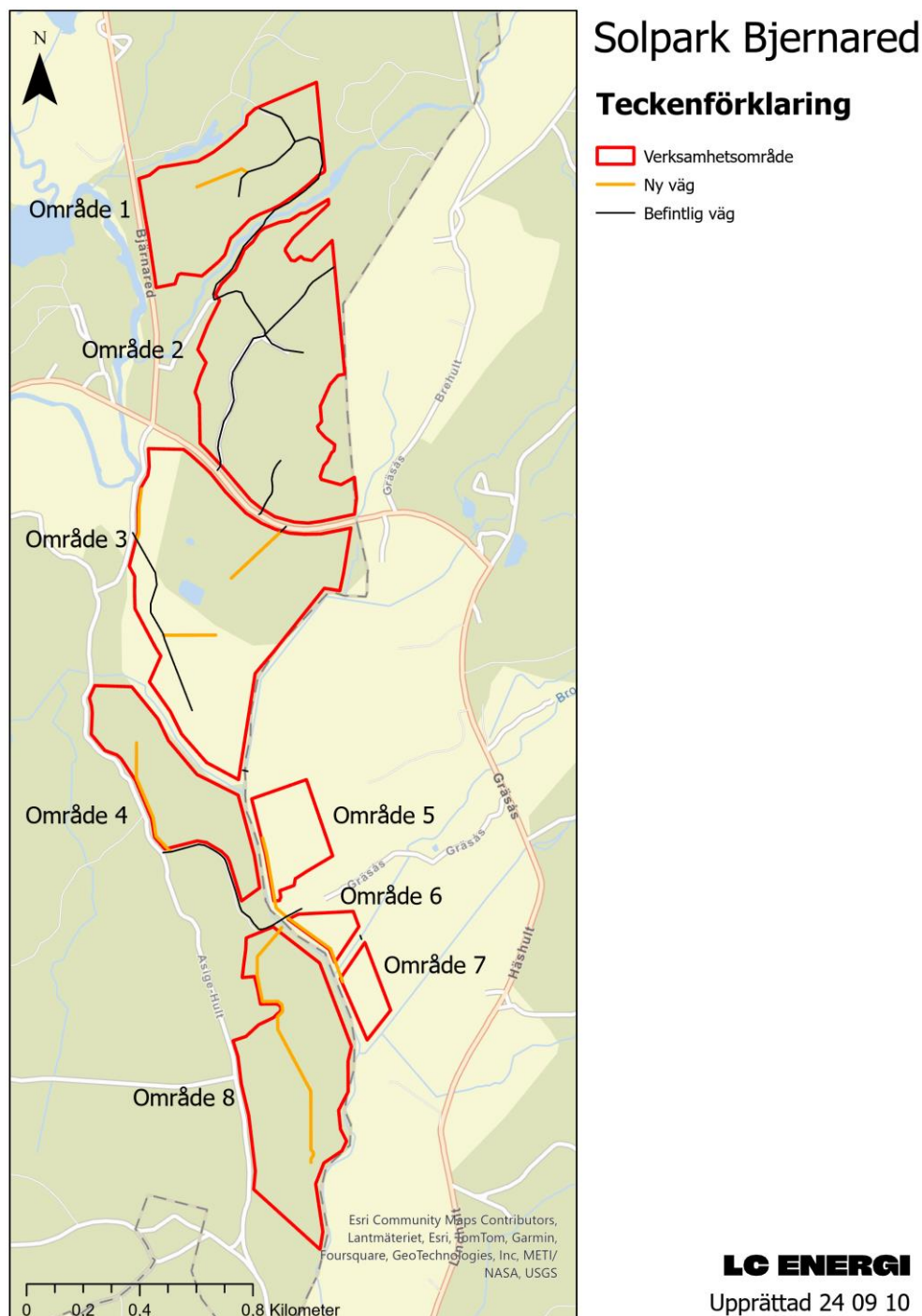
Figur 13. Placering av nya och befintliga vägar inom verksamhetsområdet (LC Energi).
