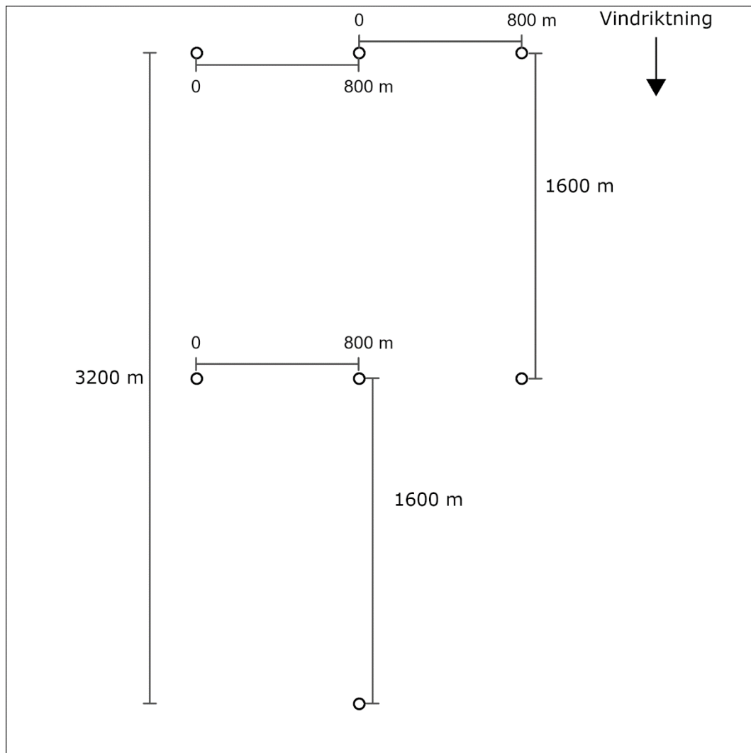
Figur 1. Exempellayout med 7 verk. Vita prickar representerar vindkraftsturbiner.
