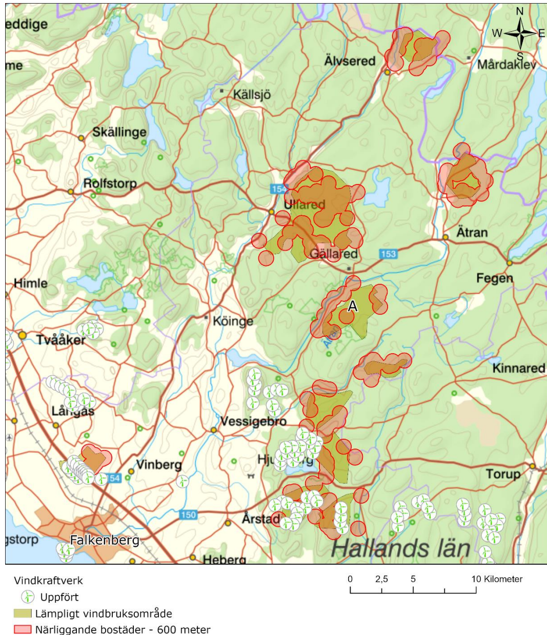
Figur 7. Utpekade vindbruksområden i Falkenbergs kommun i jämförelse med befintliga vindkraftverk samt ett konservativt skyddsavstånd om 600 meter från närläggna bostäder.
