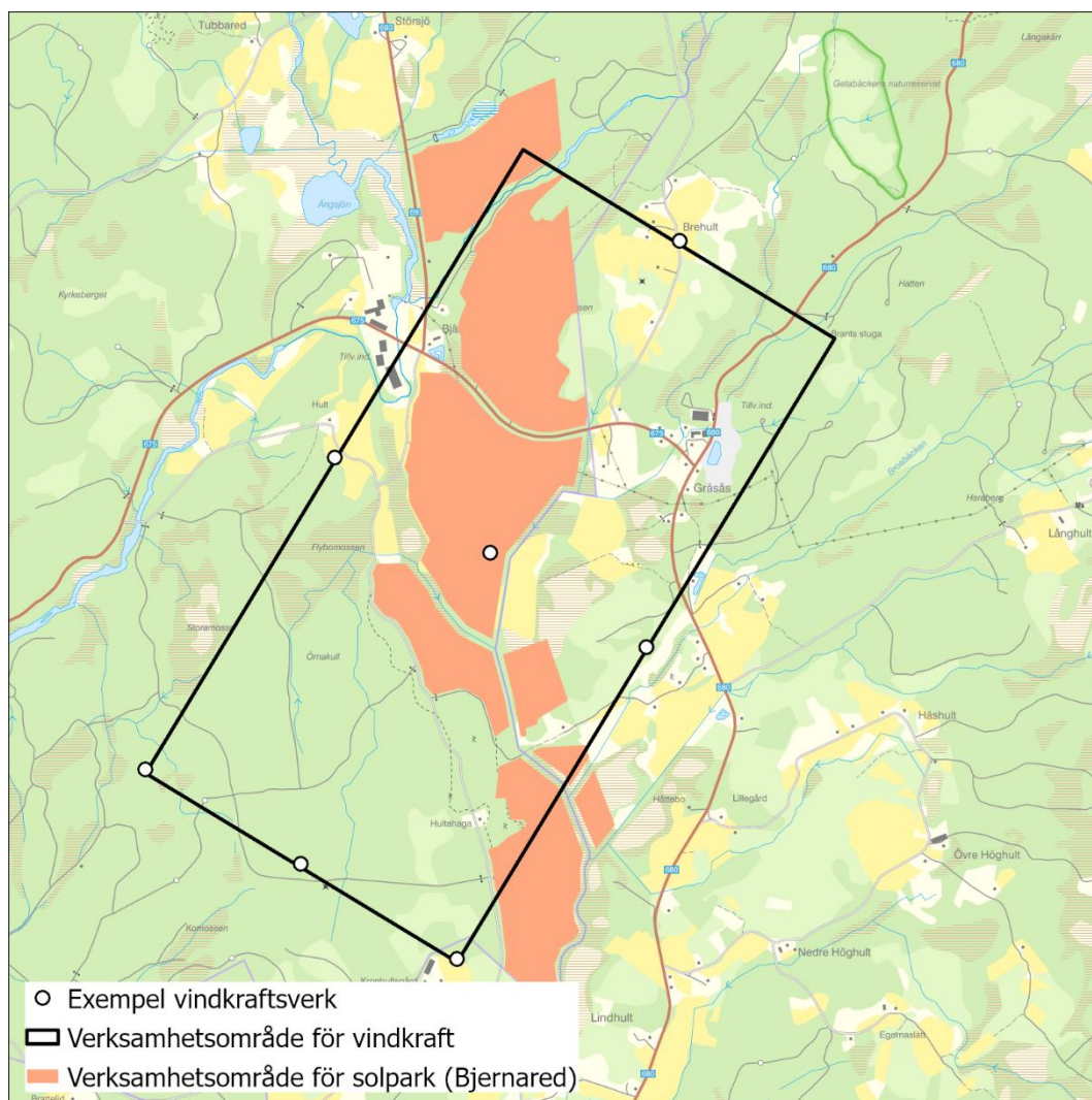
Figur 2. Exempellayout med Bjernerad verksamhetsområde i bakgrunden.
