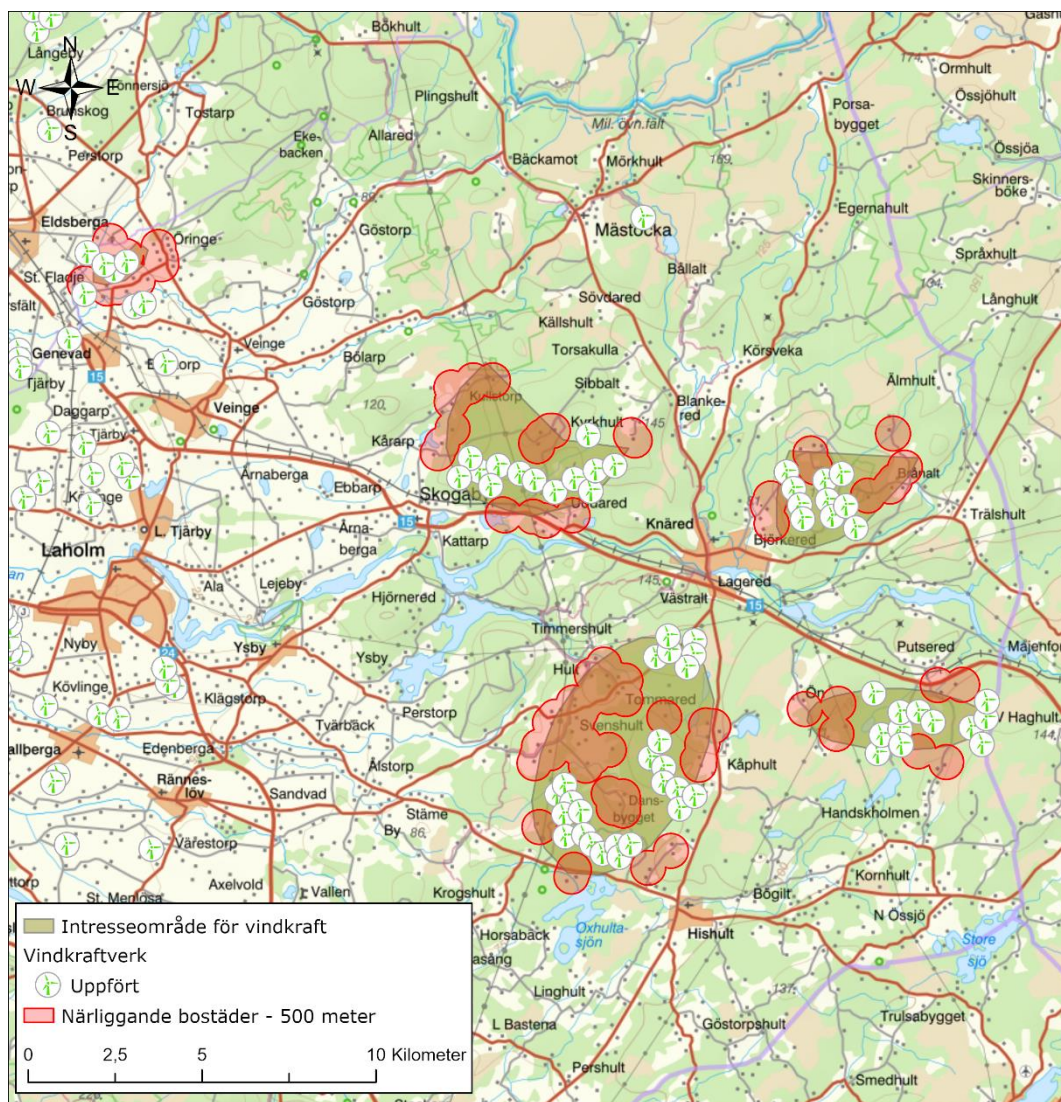
Figur 14. Vindkraftsområde i Laholms kommun med skyddsavstånd och befintliga vindkraftsverk.
